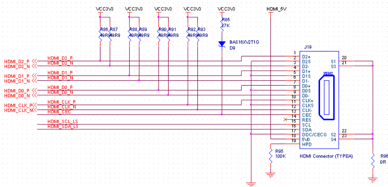
图 3-8-1 HDMI 接口设计原理图
