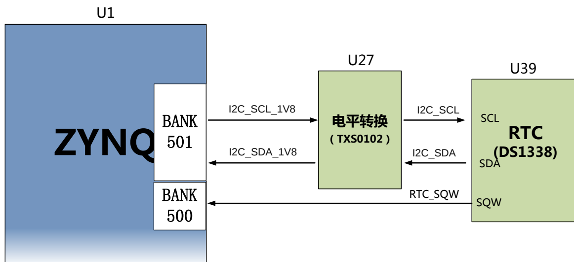
图 3-12-1 DS1338 原理图
